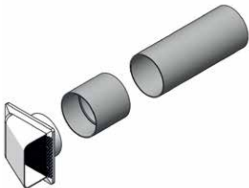
Paloilmaliitântä standard: sokkelin/seinän läpivientisarja IA-AIR00-000 putki Ø 100mm, pit. 250mm kaulus pit. 100mm
