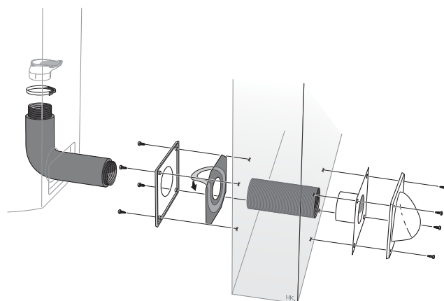
Paloilmaliitântä: sokkelin/seinän läpivientisarja, kondenssieriste & putki IA-80655-200
