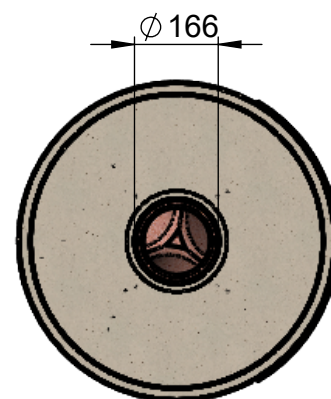
SECTION D-D
