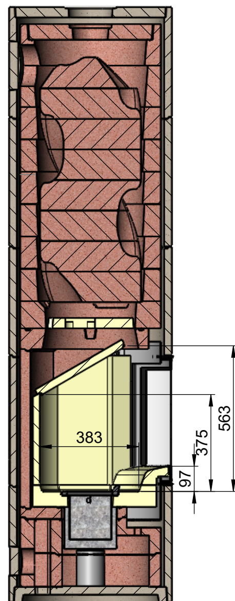
SECTION D-D
