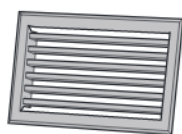
Lämminilmaritilä 150cm 2 asennusaukon koko 255x130mm, läpäisyalue 150cm 2 musta (198170) harmaa (198169)
