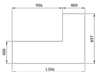
Contura 41-sarja ilman penkkiä, 1-osainen
