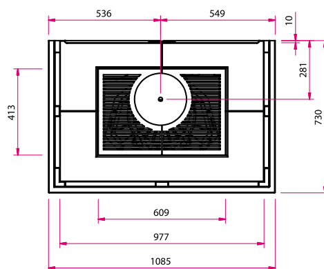
Draufsicht M 1:25
